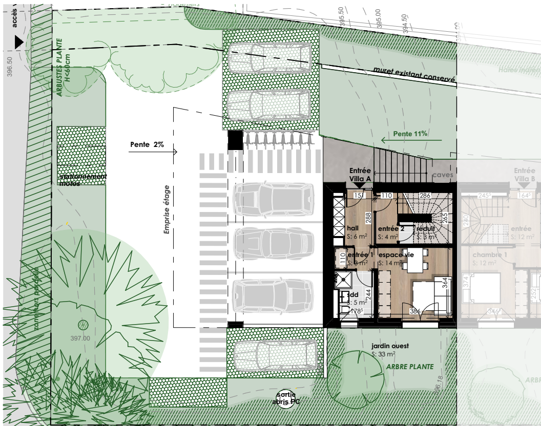
REZ DE JARDIN - VILLA B
